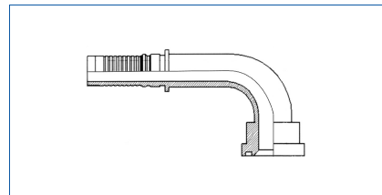
Code 61 Flange 90° Interlock
