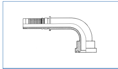
Code 61 Flange 90° Interlock
