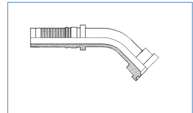
Code 61 Flange 45° Interlock
