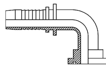
Code 61 Flange 90°
