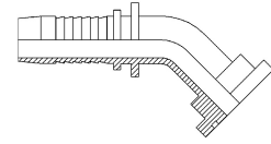
Code 61 Flange 45°
