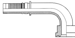
Code 62 Flange 90°
