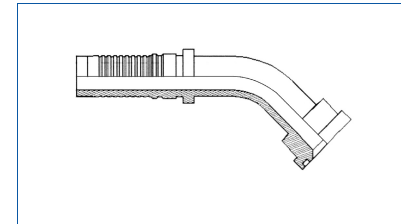
Code 61 Flange 45° Interlock
