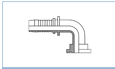
Code 62 Flange 90°
